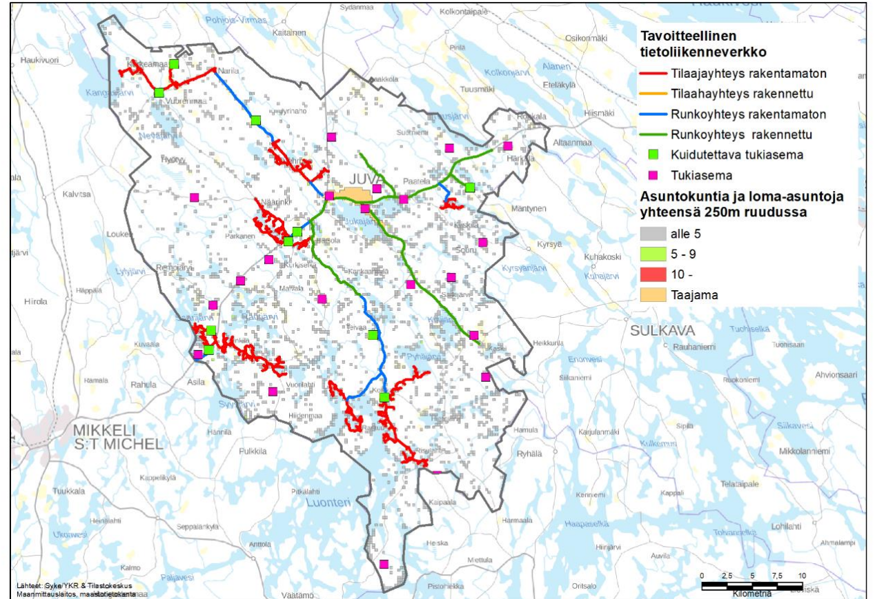
Juvan tavoitteellinen tietoliikenneverkko, luonnos
