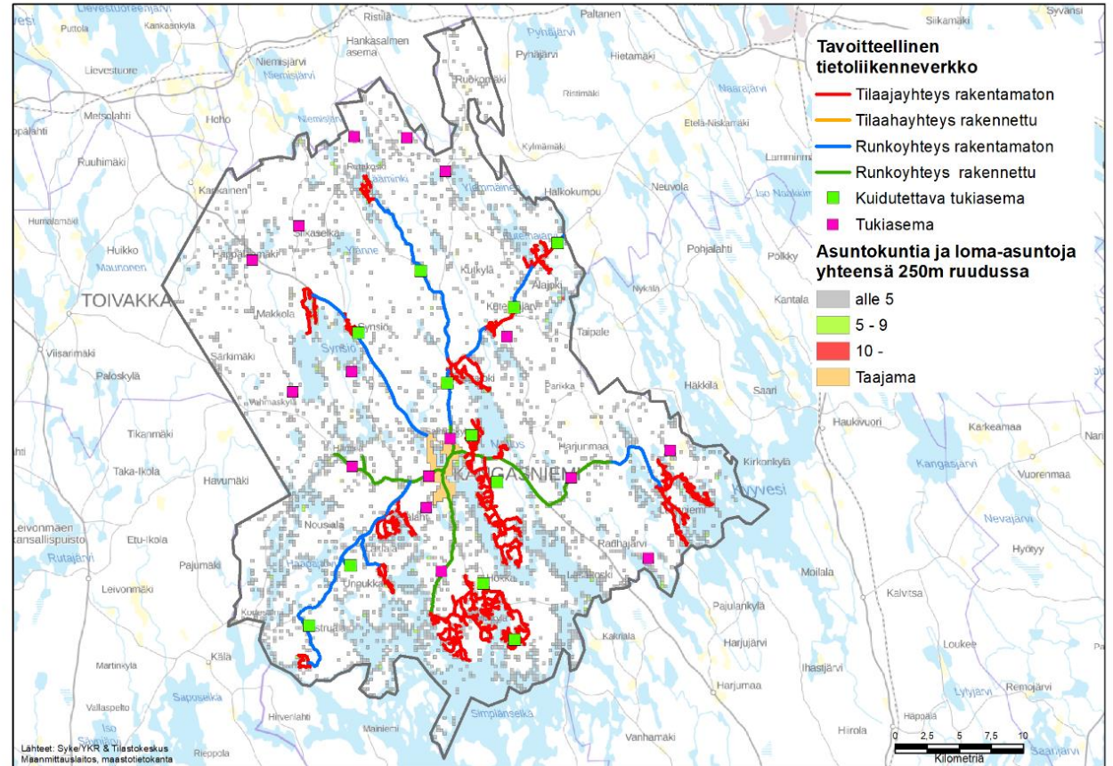
Kangasniemen tavoitteellinen tietoliikenneverkko, luonnos
