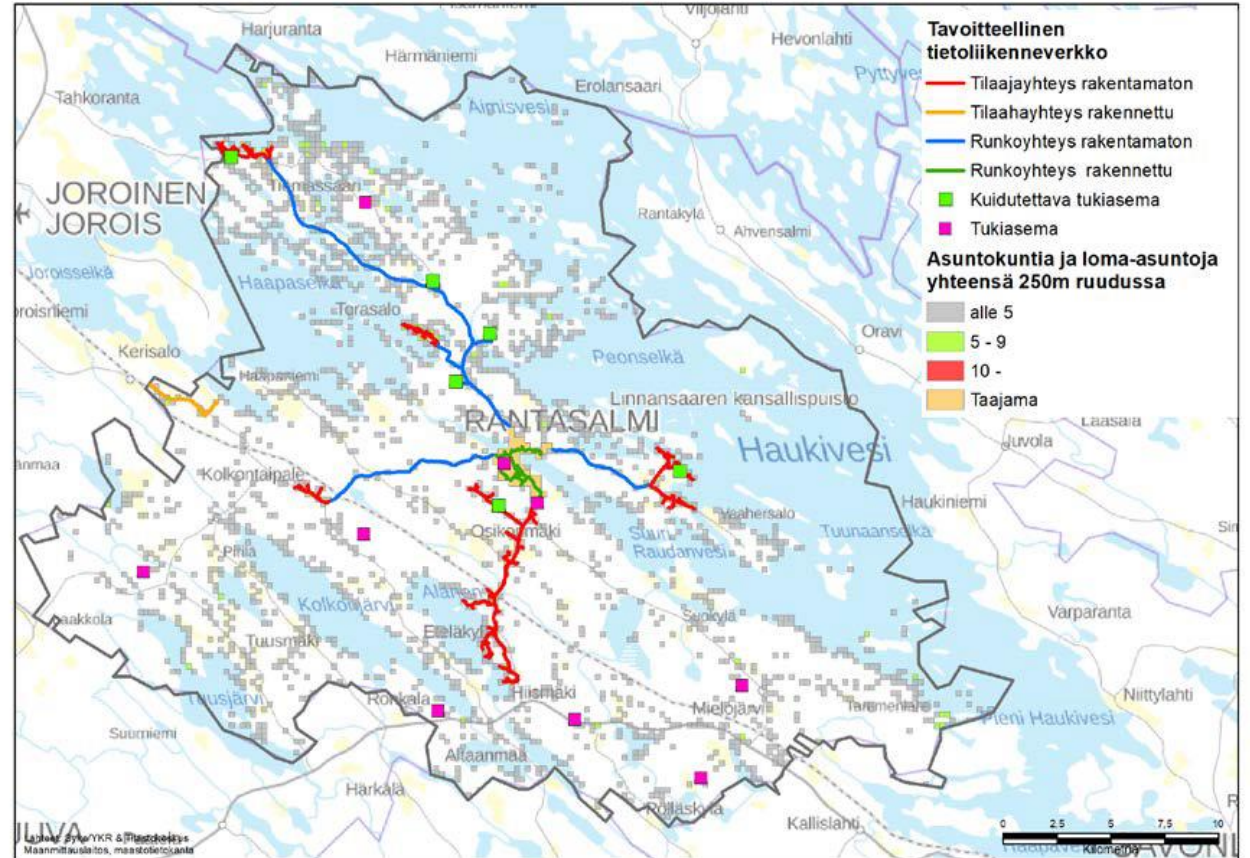
Rantasalmen tavoitteellinen tietoliikenneverkko, luonnos
