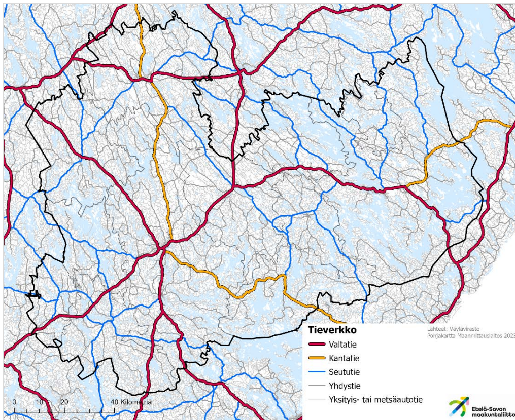
Kuva 18. Tieverkko
