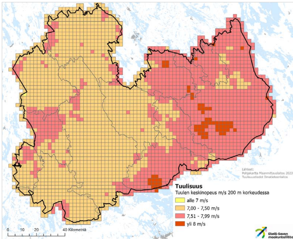
Kuva 19. Tuulen nopeus 200 metrin korkeudessa. (Suomen tuuliatlas 2009)
